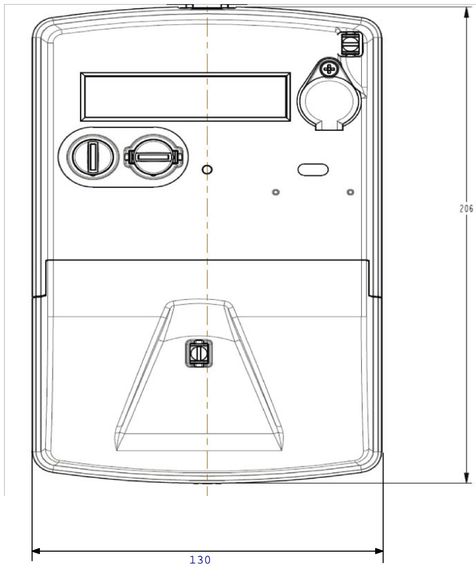
Slika 11: izmjere brojila ACE431P2 sa poklopcem priključnice
