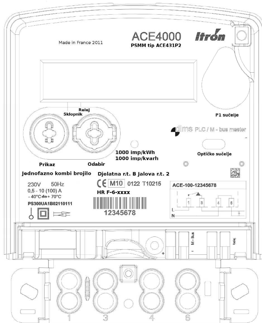
Slika 12: natpisna ploča jednofazno g brojila ACE431P2
