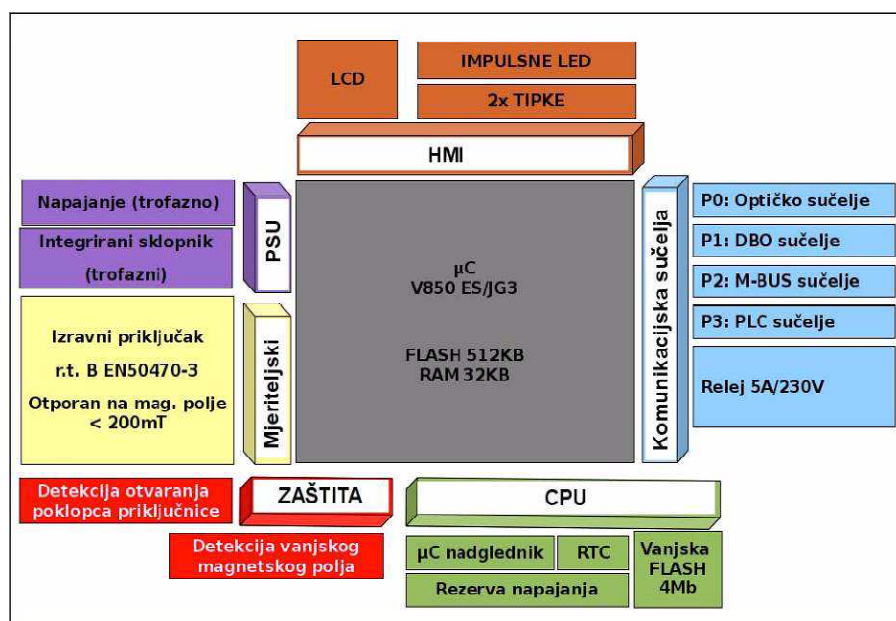
Slika 2: blok shema brojila
