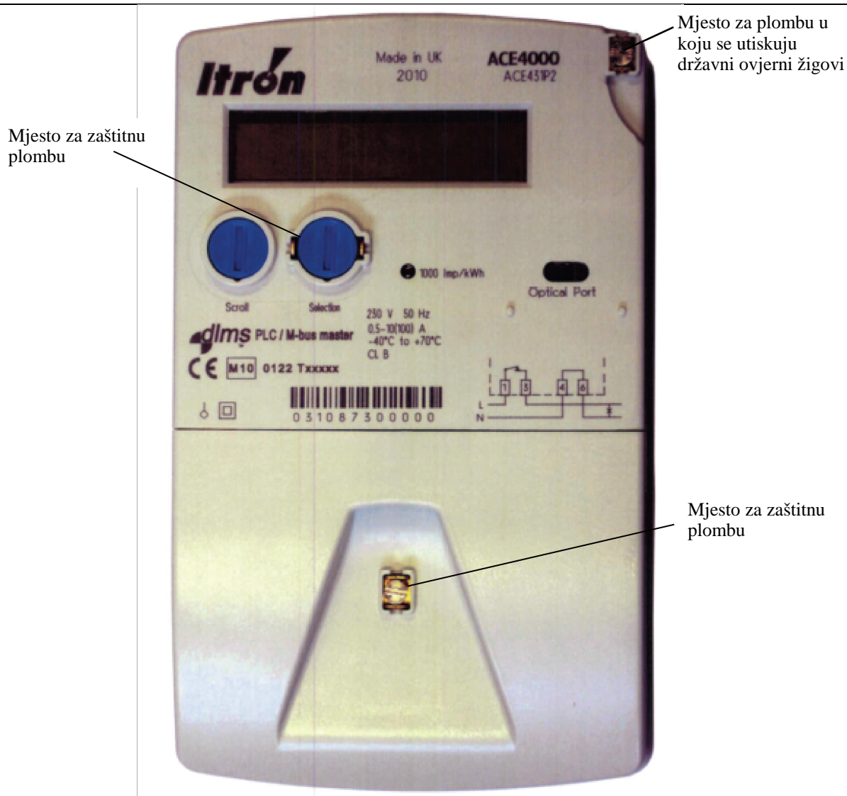
Slika 8: brojilo ACE431P2 sa označenim mjestima za plombiranje
