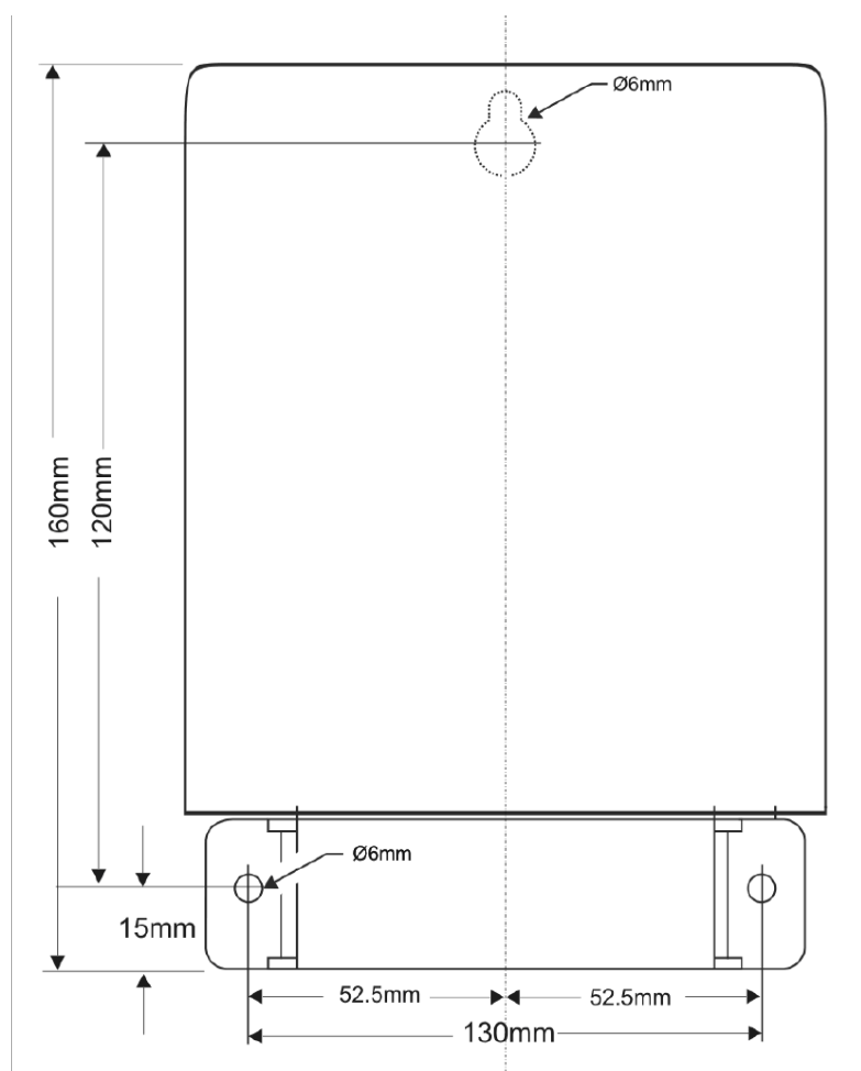
Slika 10: izmjere brojila ACE431P2 bez poklopca priključnice
