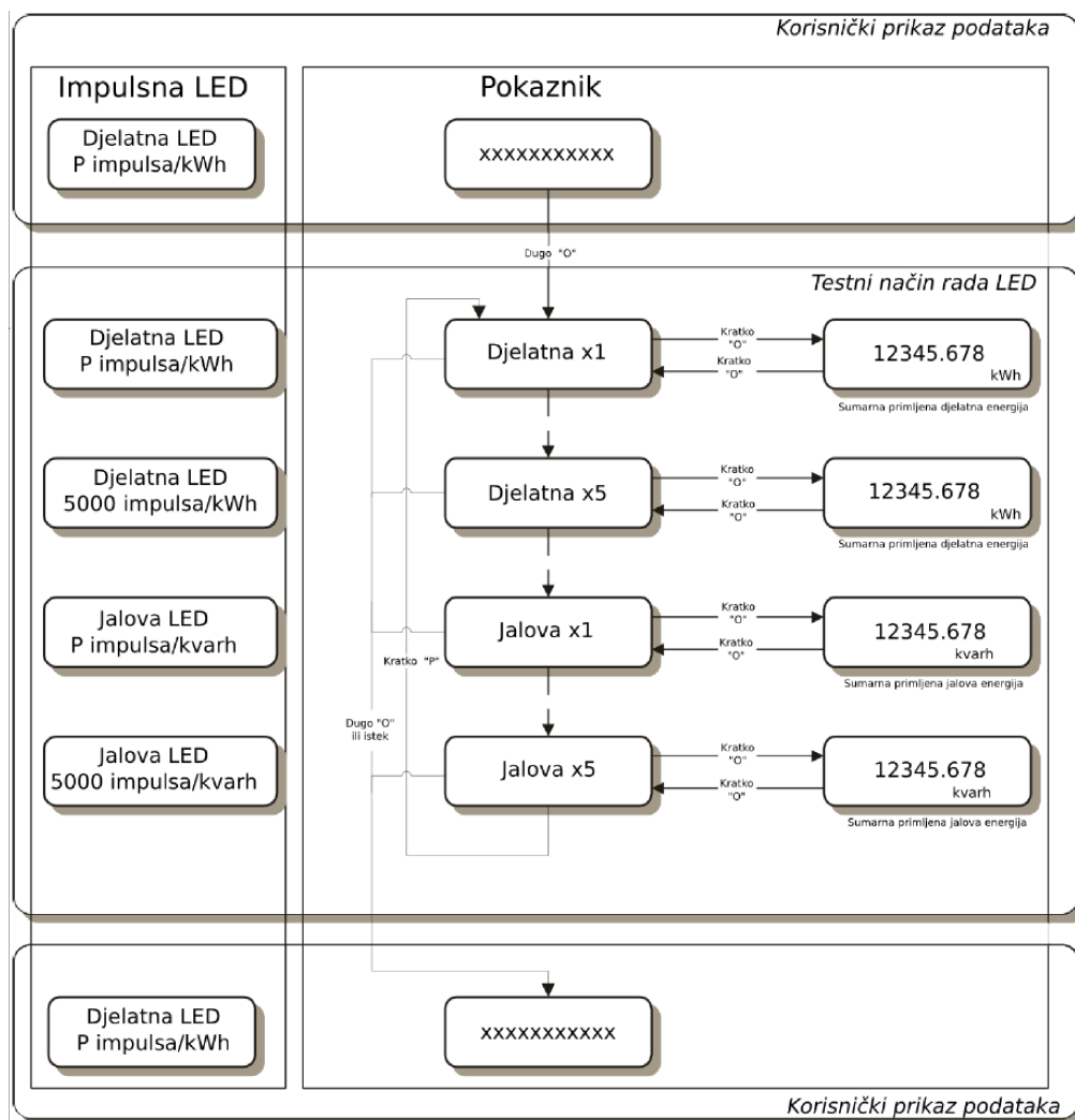
Slika 6: prikaz način rada pokaznika u testnom načinu rada
